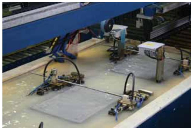
Obr.2: Skúška tesnosti
