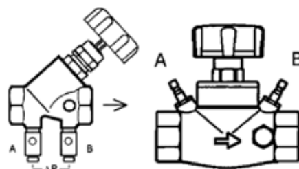
Obr. 6: Regulačné armatúry
